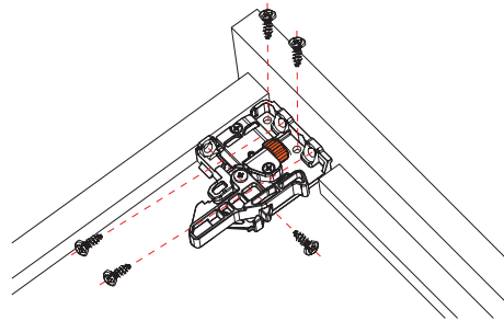
Fije el dispositivo de bloqueo en el fondo del cajón. Fix the locking device onto the drawer bottom.
