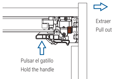
Para extraer el cajón pulse el gatillo y saque el cajón. For removal, hold the handle and pull out the drawer.
