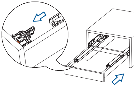
Coloque la parte inferior del cajón en las guías y empuje. Lay the drawer bottom onto the slide the push the drawer into the cabinet.
